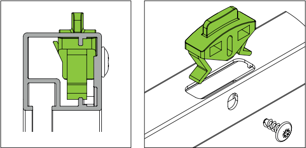
PROWADNIK G/D MINI RAM | GUIDE G/D MINI RAM
